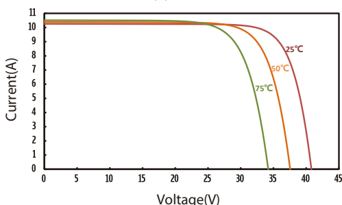
JT330SIh(B) 不同温度下的IV曲线
